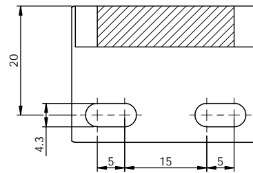
剖面 K-K
